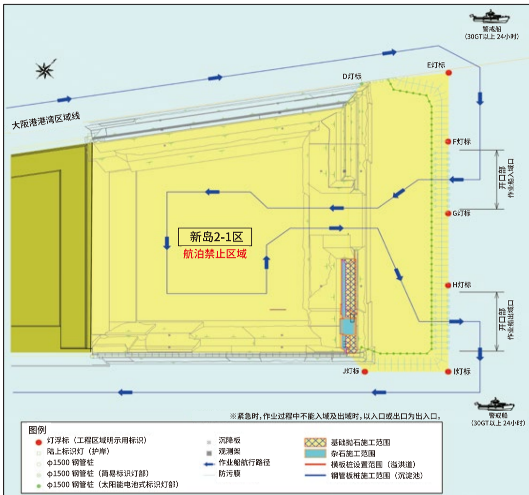
施工平面图（航泊禁止区域图）
